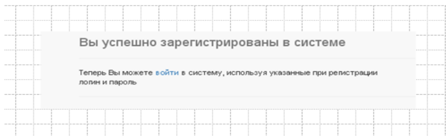
Рисунок 6 – Успех регистрации
