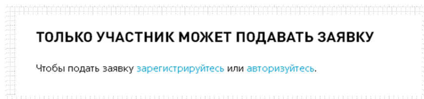
Рисунок 3 – Возможный результат
