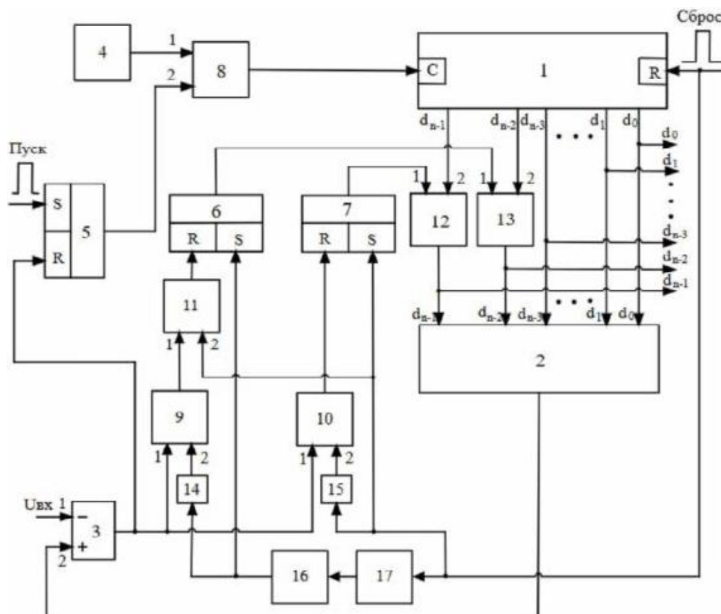
Рис.1 – Функциональная схема последовательного преобразователя напряжение-код
